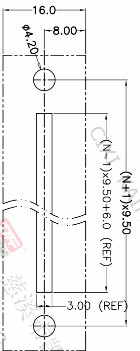
P.C.B. LAYOUT
