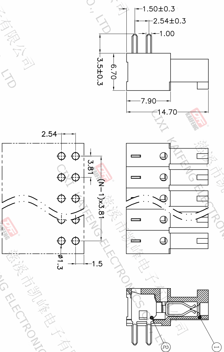
P.C.B.LAYOUT
